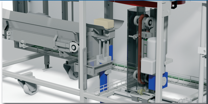
Detailansichten doppelter Absenker
